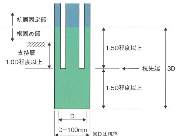
根固め部築造図
