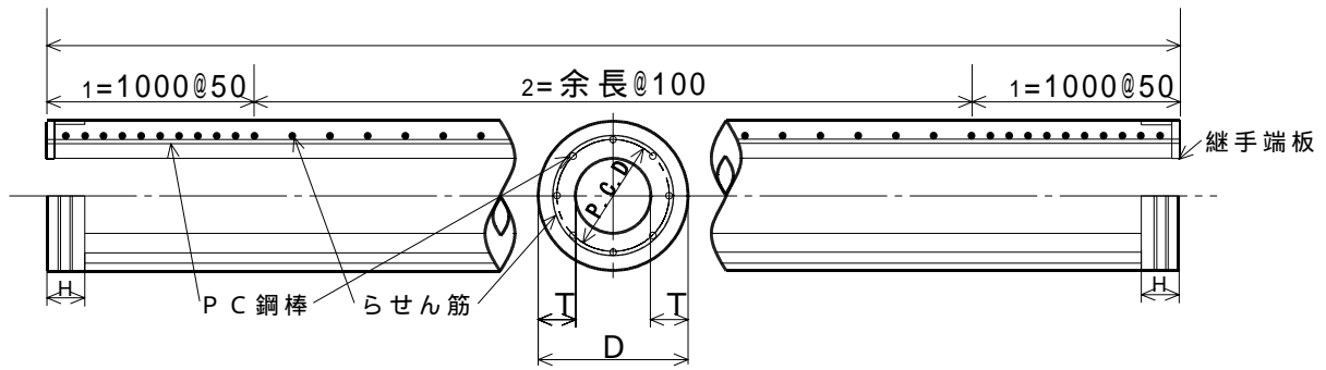
図 - 1 マナックNACパイル標準構造図
